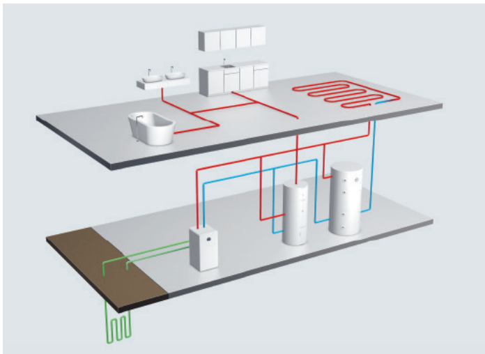
Schematische Darstellung von Raumheizung und Warmwasseraufbereitung bei einem Einfamilienhaus mit der Sole-Wasser-Wärmepumpe Bosch CS7800i 8 LW.
